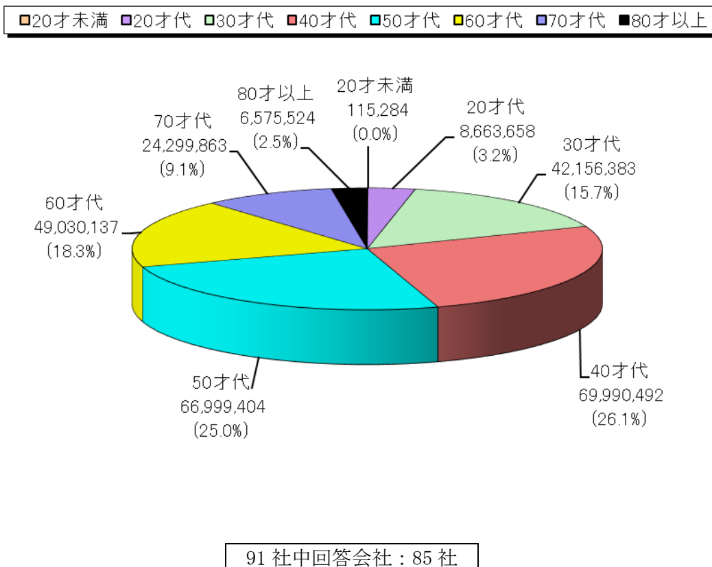
図-8 株式等(信用取引)の年代別売買代金及び売買代金比率
