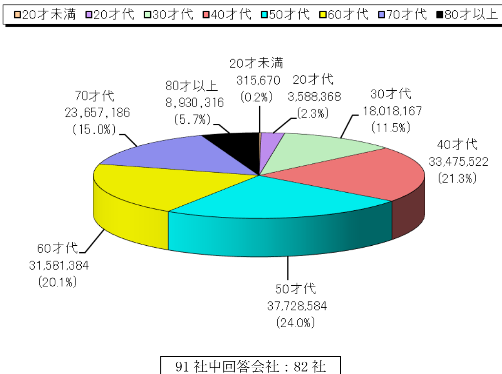
図-7 株式等(現物取引)の年代別売買代金及び売買代金比率
