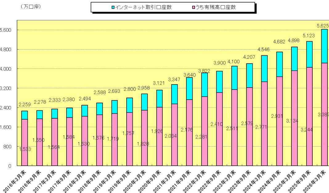
図-2 インターネット取引口座数
