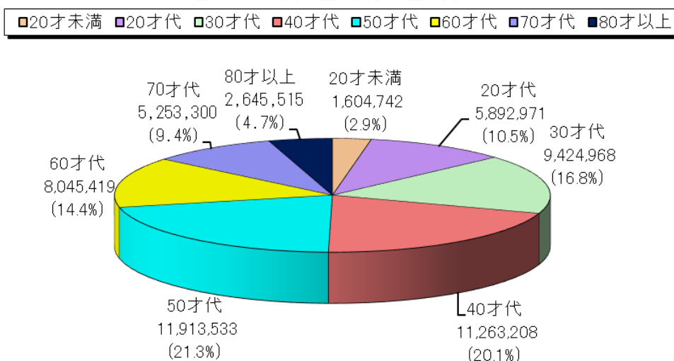
図-3 年代別口座数及び口座数比率
